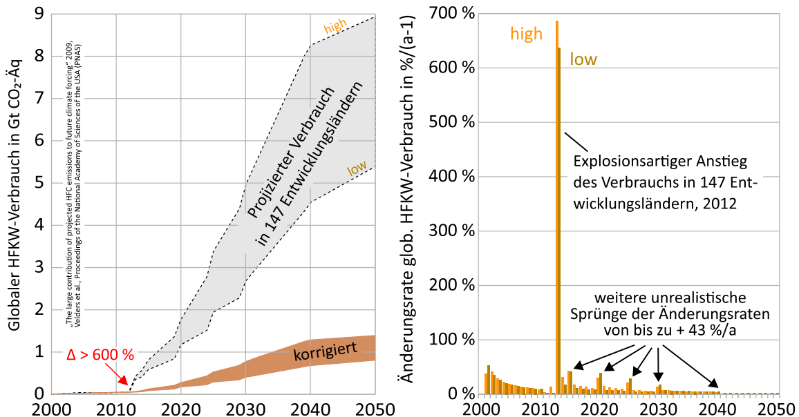
Globaler, projizierter Verbrauch von HFKW, zugehörige Änderungsraten und Korrektur
